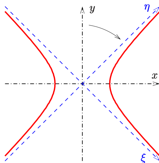
▲ Figuur 1: Afbeelding van een hyperbool (Maker: Ag2gaeh, Creative Commons Attribution-Share Alike 4.0 International)
