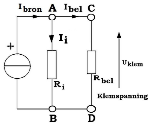
Niet-ideale stroombron
