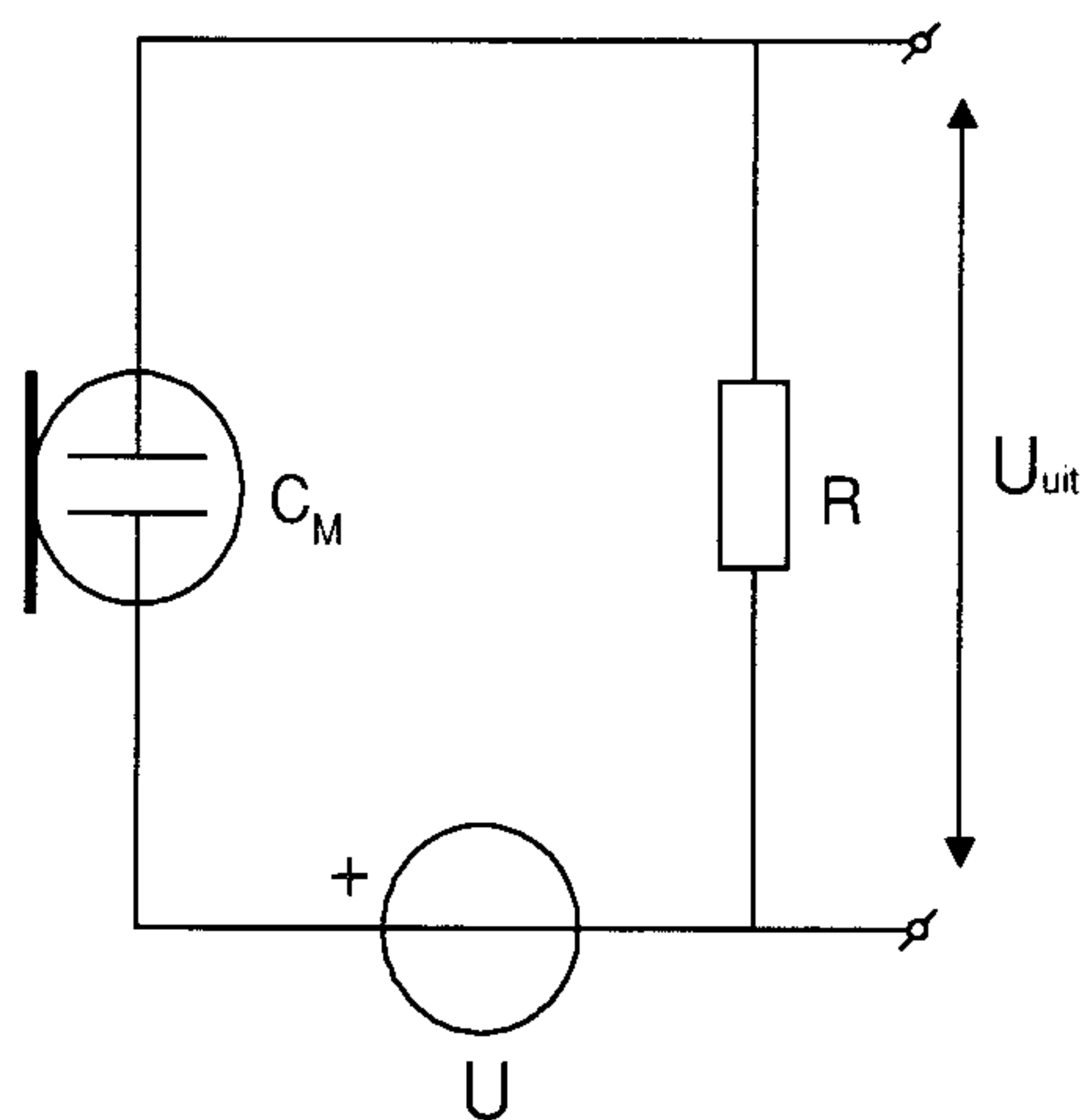
Figuur 6-2 Een condensatormicrofoon schakeling
