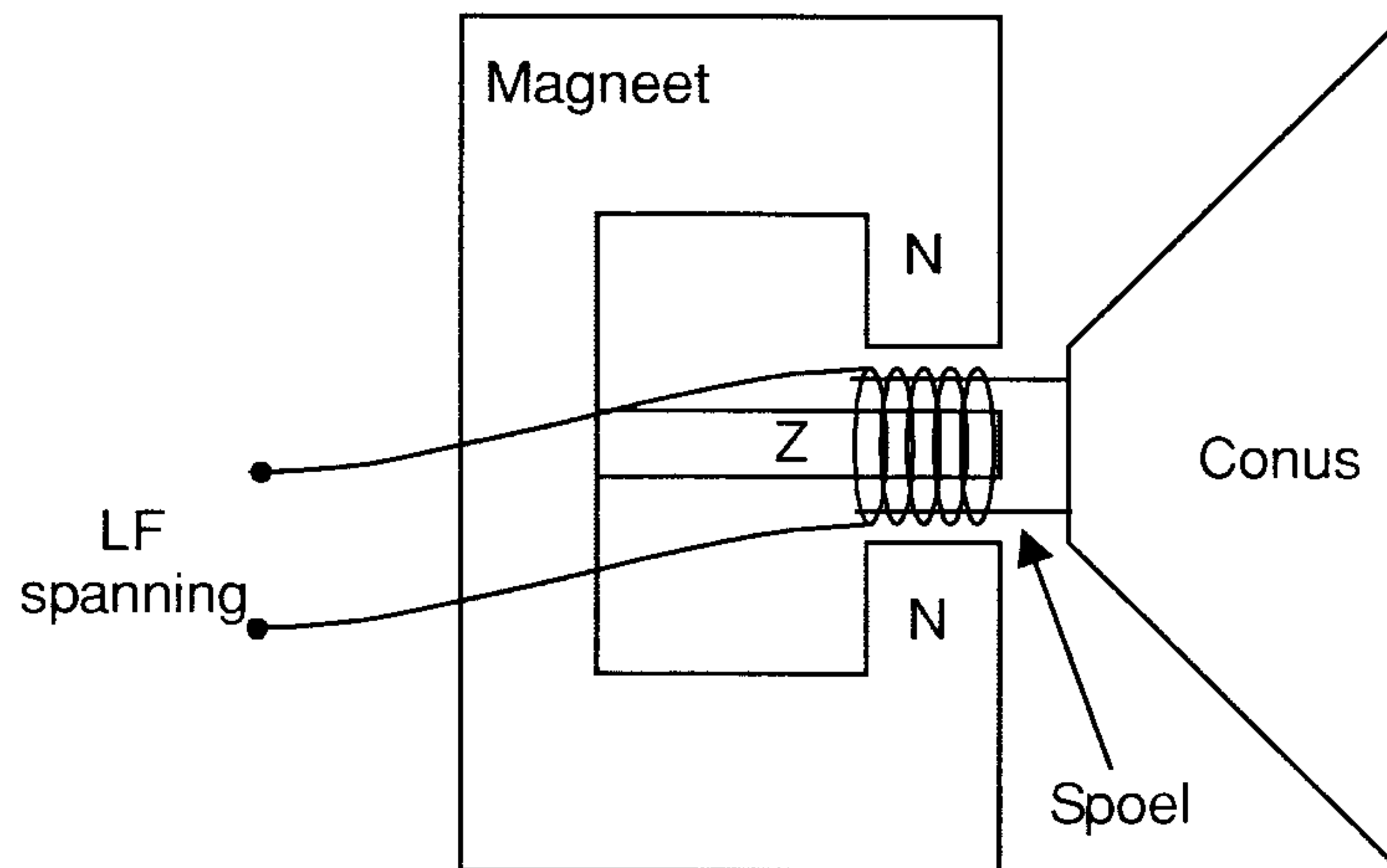
Figuur 6-5 Een luidspreker voor hoog vermogen
