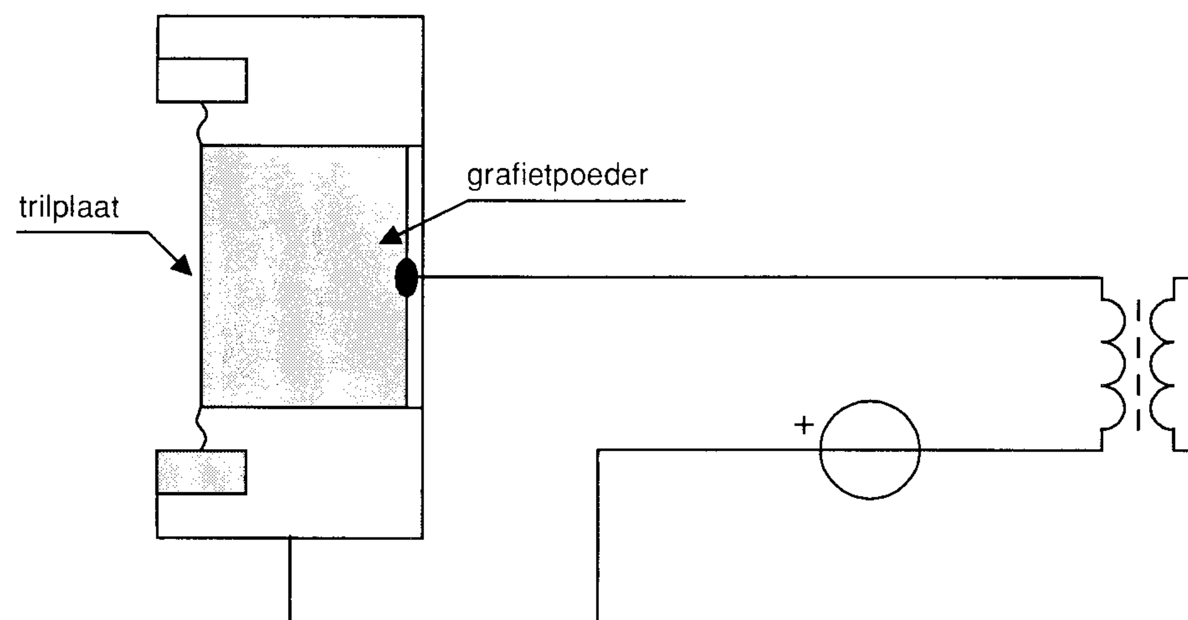
Figuur 6-1 Een koolmicrofoon.
