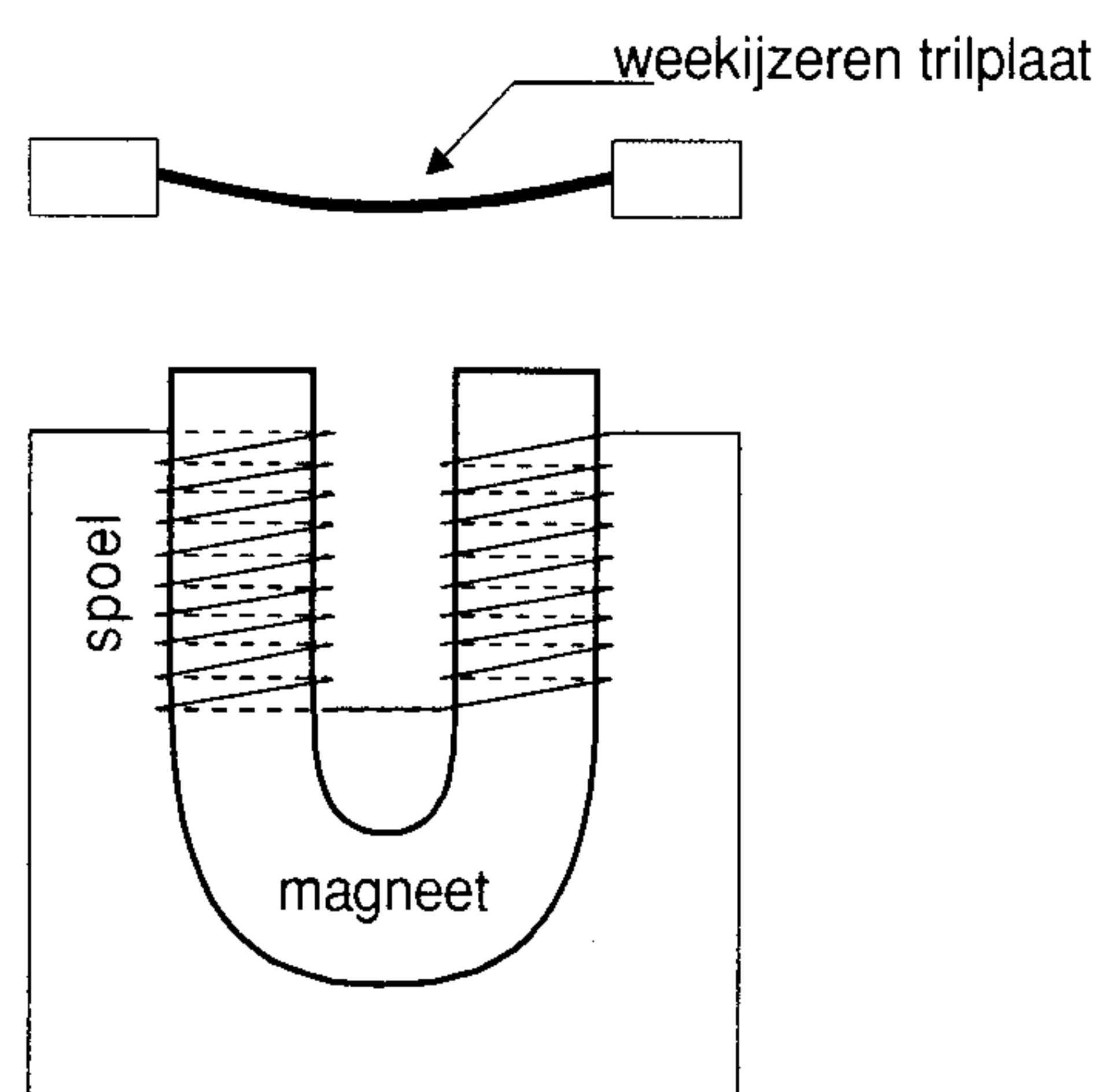
Figuur 6-3 Een elektro-dynamische luidspreker.
